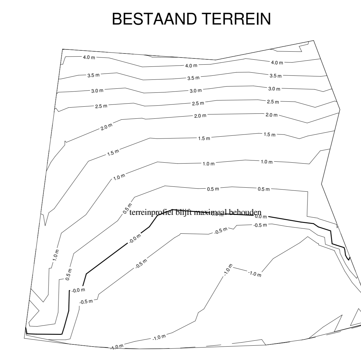
2 Hoogtemeting terrein 1 : 250
