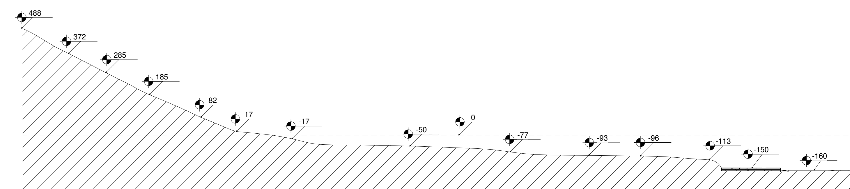
3 Bestaand terreinprofiel 1 : 100
