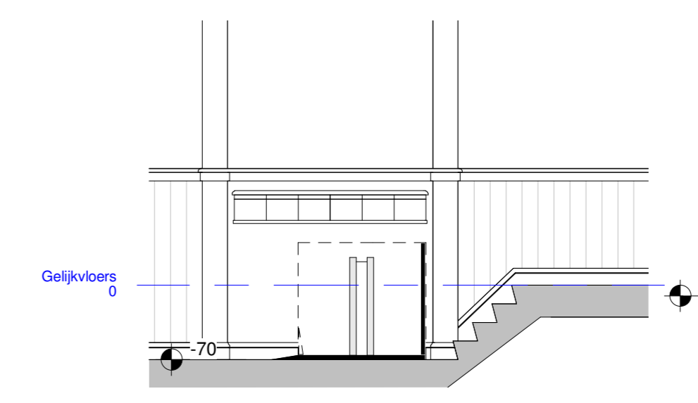
6 vert plateaulift B 1 : 50
