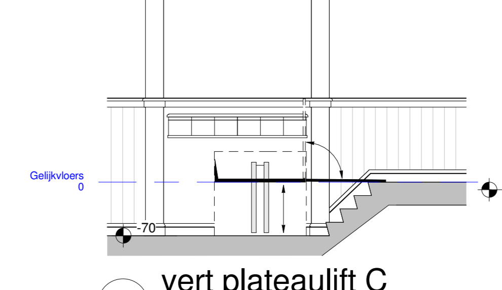
7 vert plateaulift C 1 : 50
